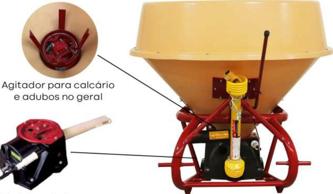
Unidade mecânica
